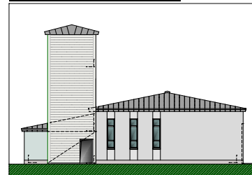
Pohled jihovýchodní (1:200)
