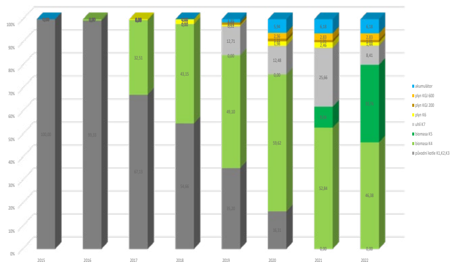
Dodávka tepla do sítě CZT dle zdroje tepla v % v letech 2015 - 2022
