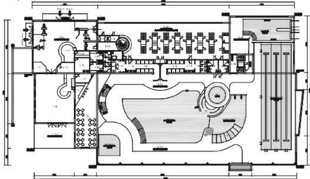
Varianta "C" : SO Krytý bazén - Řešení vztahů a návaznosti Půdorys 1.NP , m 1:100
