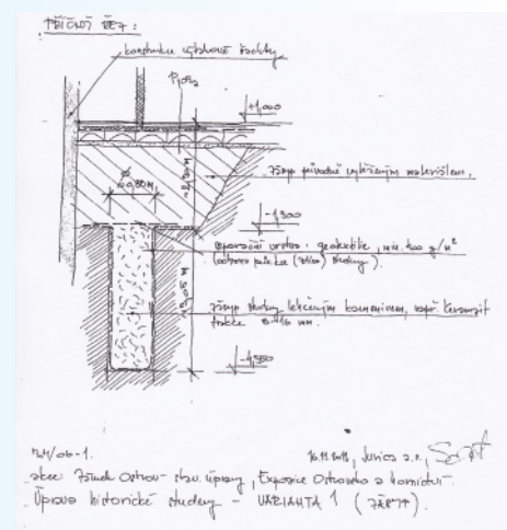
Průřez studnou
